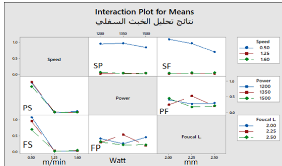
شكل 8: التأثيرات المشتركة للمعاملات على تكون الخبث
