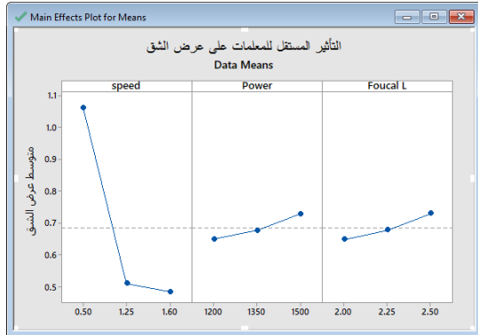
شكل 1: عرض الشق المقابل لمستويات المعاملات
