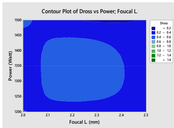
شكل 12: التأثير المشترك للقدرة والبعد البؤري على معدل تكون الخبث.
