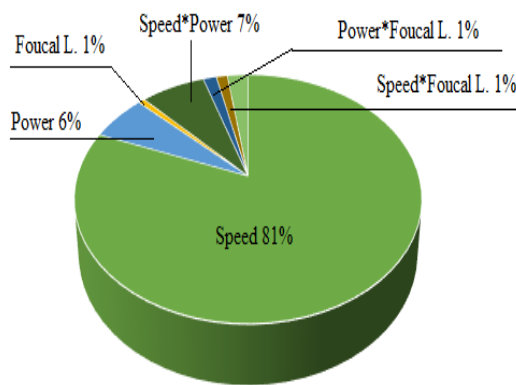
شكل 15: نسب تأثير معلمات العملية
