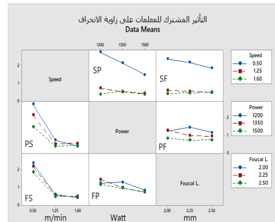
شكل 14: التأثيرات المشتركة للمعلمات على زاوية الانحراف
