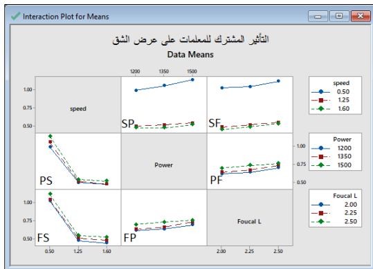
شكل 2: التأثيرات المشتركة للمعاملات على عرض الشق
