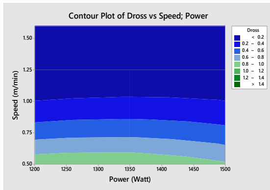
شكل 10: التأثير المشترك للسرعة والقدرة على الخبث
