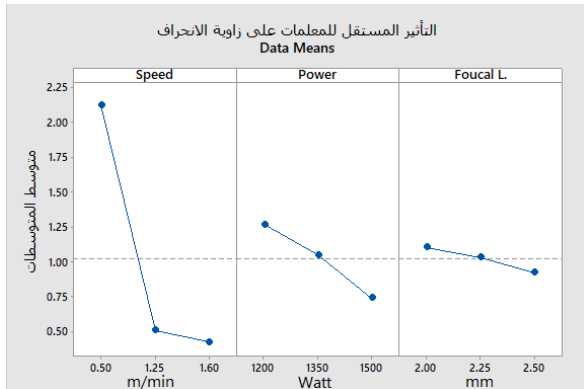
شكل 13: زاوية الانحراف المقابلة لمستويات المعلمات
