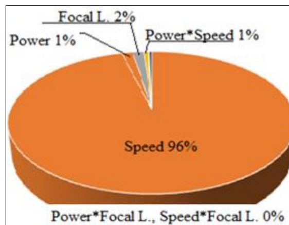
شكل 3: نسب تأثير معلمات العملية على عرض الشق.
