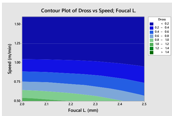
شكل 11: التأثير المشترك للسرعة والبعد البؤري على معدل تكون الخبث
