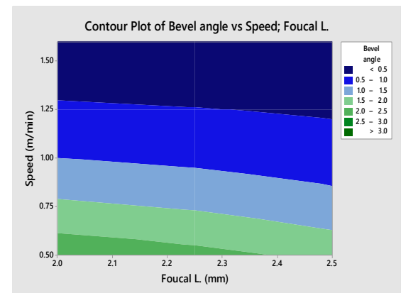
شكل 17: التأثير المشترك لسرعة القطع والبعد البؤري
