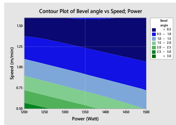
شكل 16: التأثير المشترك لسرعة القطع والقدرة
