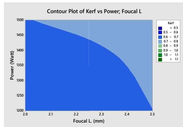
شكل 6: التأثير المشترك للقدرة والبعد البؤري.
