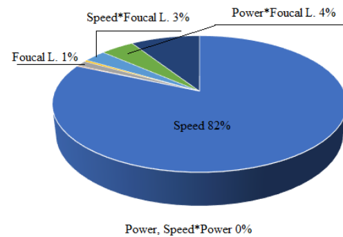
شكل 9: نسب تأثير معلمات العملية على تكون الخبث
