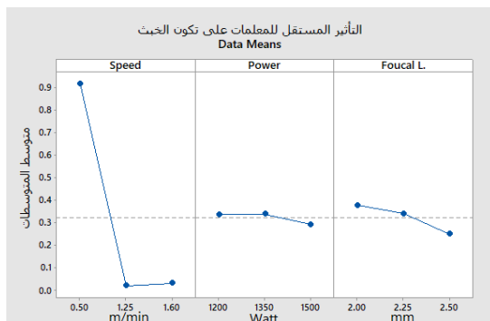
شكل 7: متوسط الخبث المقابل لمستويات معلمات العملية
