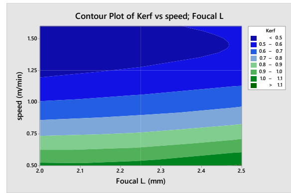
شكل 5: التأثير المشترك لسرعة القطع والبعد البؤري.
