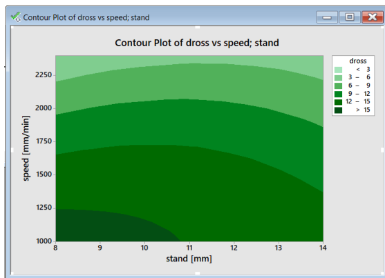
شكل 18: التأثير المشترك لسرعة القطع وارتفاع الفوهة على معدل الخبث.
