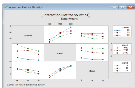
شكل 6: مخطط مؤشر (S/N ratio) للتأثيرات المشتركة للمعاملات على عرض الشق.
