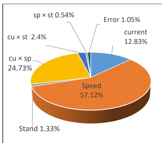
شكل 15: نسب تأثير معلمات العملية الأساسية والمشاركة على معدل الخبث.
