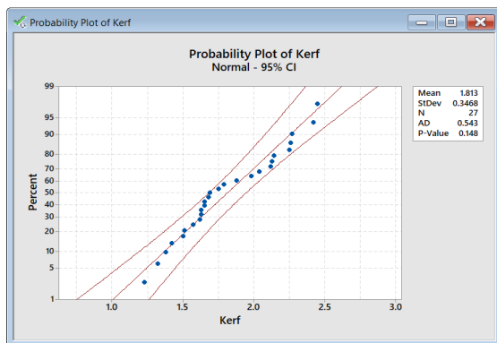
شكل 4: توزيع بيانات تأثير المعلمات على عرض الشق.
