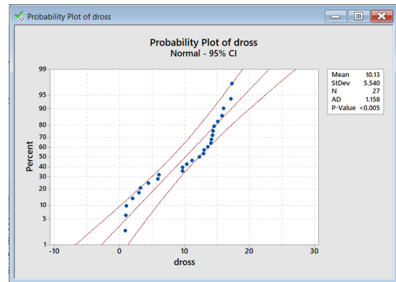
شكل 12: توزيع بيانات تجربة معدل تكون الخبث.
