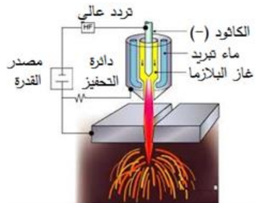
شكل 1: مكونات ومفهوم عملية القطع بالبلازما.
