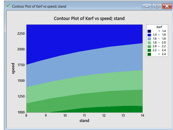
شكل 10: التأثير المشترك لسرعة القطع وارتفاع الفوهة.
