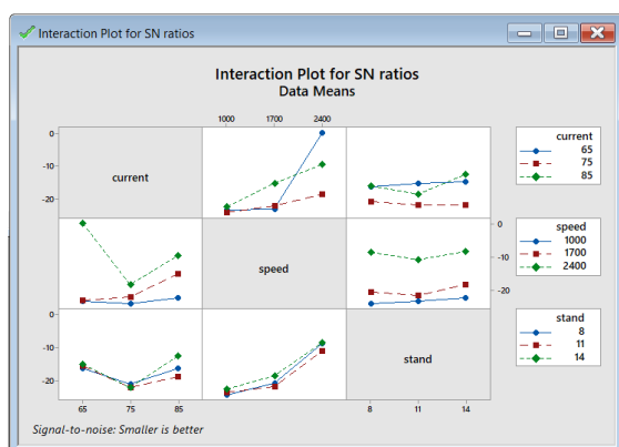
شكل 14: مخطط مؤشر (S/N ratio) للتأثيرات المشتركة على معدل تكون الخبث.
