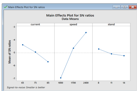
شكل 5: مخطط مؤشر (S/N ratio) للتأثيرات المستقلة على عرض الشق
