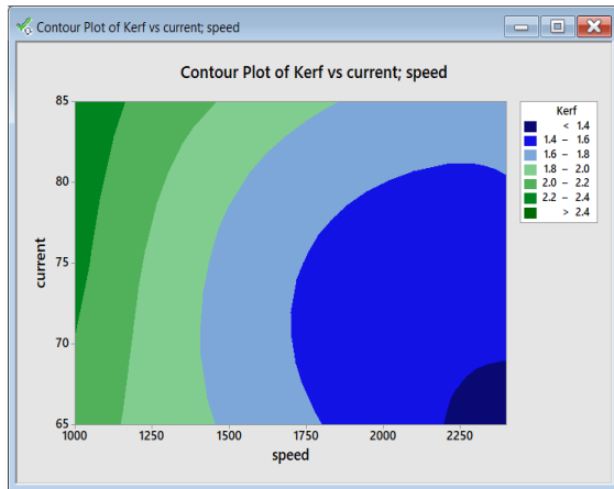
شكل 8: التأثير المشترك لشدة التيار وسرعة القطع.
