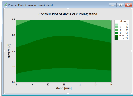
شكل 17: التأثير المشترك لشدة التيار وارتفاع الفوهة على معدل الخبث.
