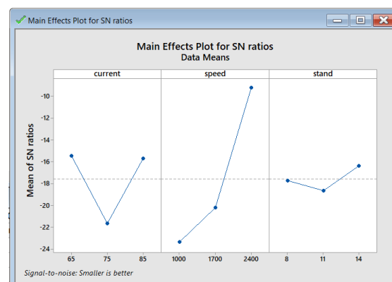
شكل 13: مخطط مؤشر (S/N ratio) للتأثيرات المستقلة على معدل تكون الخبث.
