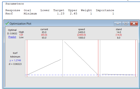
شكل 11: نتائج عملية التحسين باستخدام (Factorial design) (القيم المثالية).
