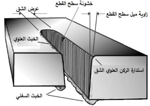
شكل 2: معايير قياس جودة عملية القطع بالبلازما [3].
