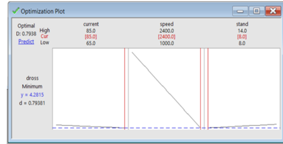
شكل 19: القيم المثالية للمعلمات وفق عملية التحسين (ت) تجربة اختبار النماذج.
