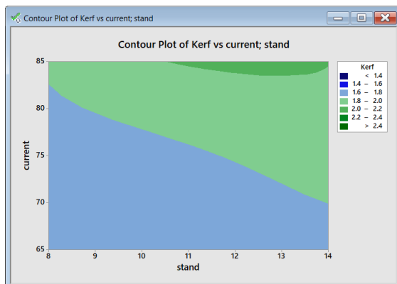
شكل 9: التأثير المشترك لشدة التيار وارتفاع الفوهة.
