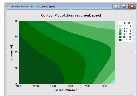
شكل 16: التأثير المشترك لشدة التيار وسرعة القطع على معدل الخبث.
