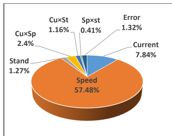
شكل 7: نسب تأثير معلمات العملية على عرض الشق.
