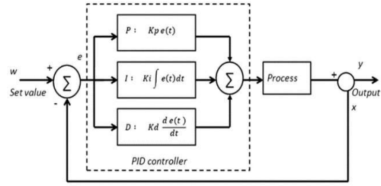
الشكل 1. حلقة المتحكم PID
