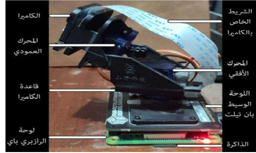
الشكل 5. أجزاء الجهاز
